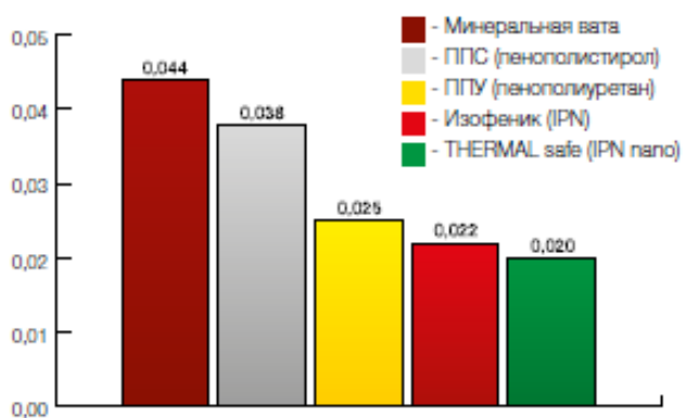
Сравнение коэффициентов теплопроводности (λ) различных изоляционных материалов используемых в сэндвич-панелях
